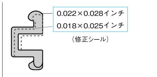
図① ブラケットの断面図
