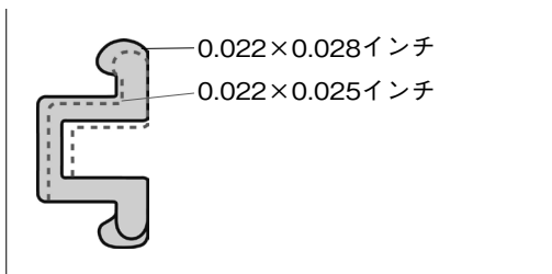
図① ブラケットの断面図
